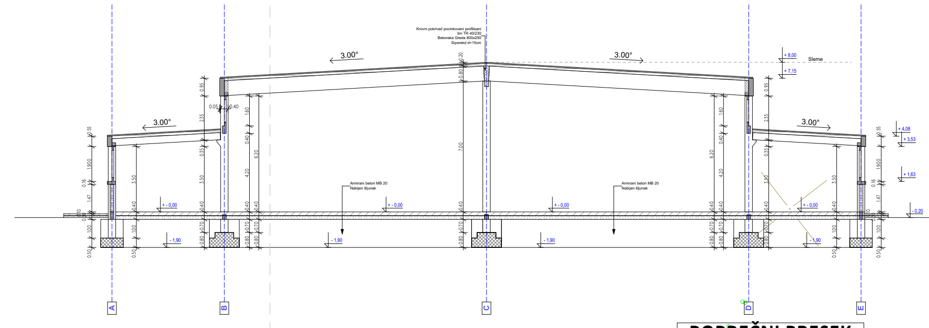
POPREČNI PRESEK
